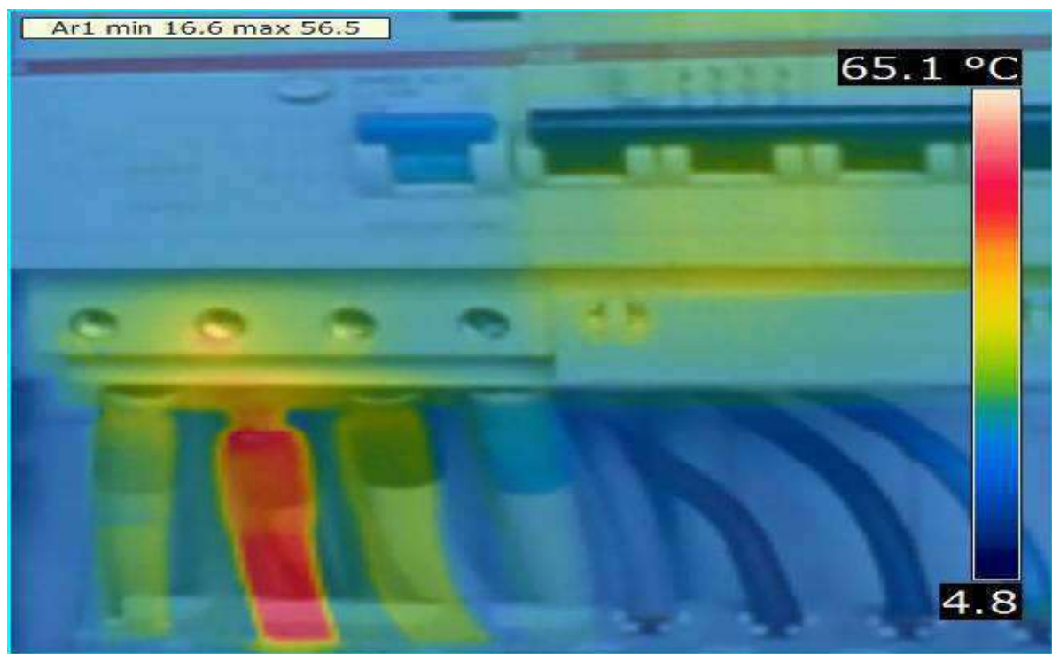
Termografia applicata ad un interruttore magnetotermico differenziale
